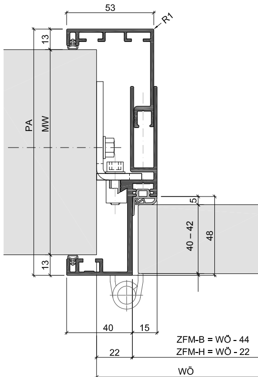
Huisserie enveloppante EUROKS
