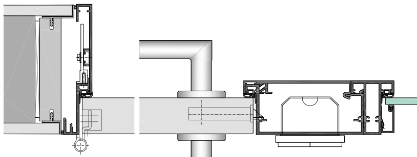
LZS avec rouleau de paumelle apparent, et panneau de porte avec module terminal de porte TTM pour boîtiers d'appareillage pour interrupteurs, prises et guidage de câbles et conduites
